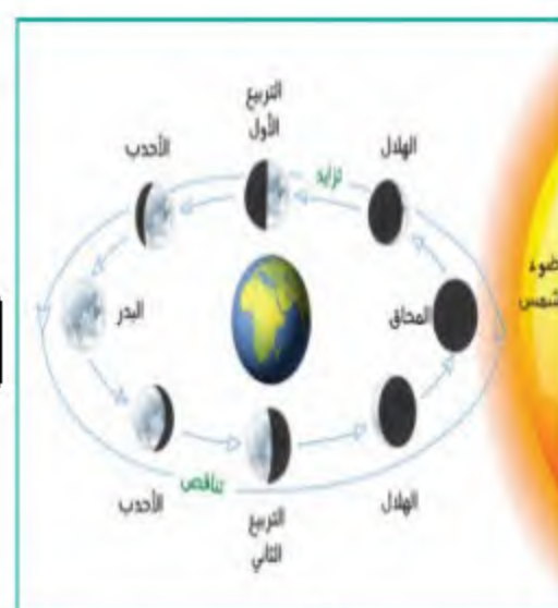
أوجه القمر
