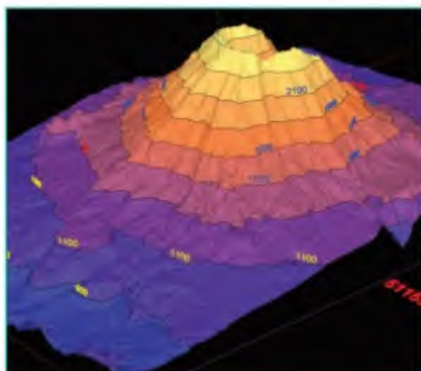
خطوط الكنتور
