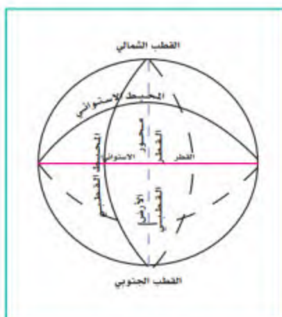
أبعاد الأرض
