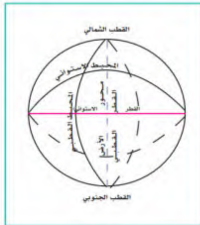
أبعاد الأرض
