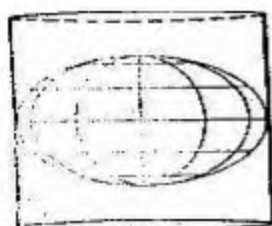
المساقط الاسطوانية
