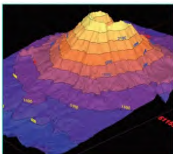
خطوط الكنتور
