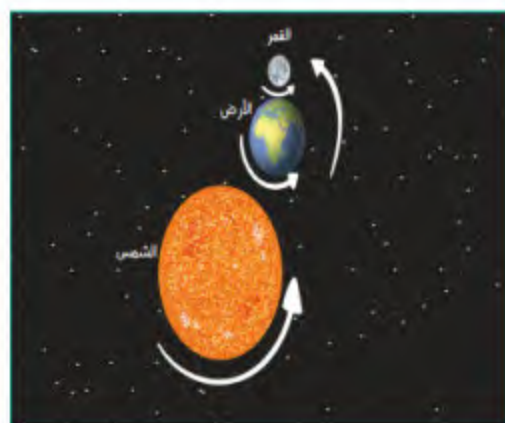
حركة الأرض
