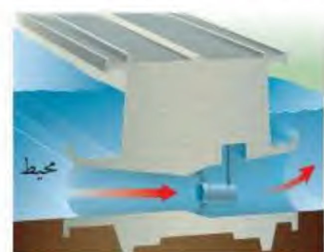
ب خلال المد تدير حركة الماء التوربين المرتبط مع المولد الكهربائي، وعند اكتمال المد تغلق البوابة لتحجز الماء خلف السد.
