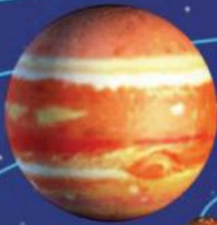
المُشْتَرِي
