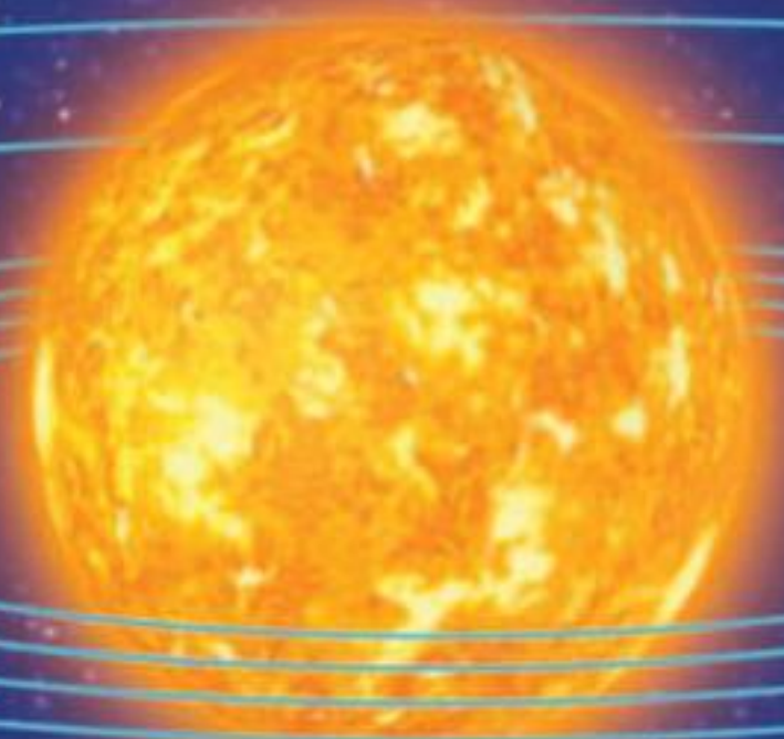
الشَّمْسُ
