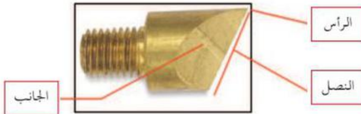
الشكل (١٦٥): الرأس الأكثر استخداماً في التحديد .
