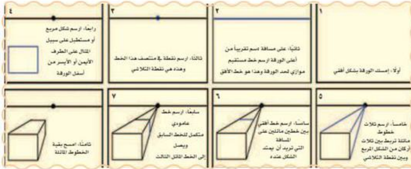
شكل (١٨): خطوات استخدام المنظور البسيط.
