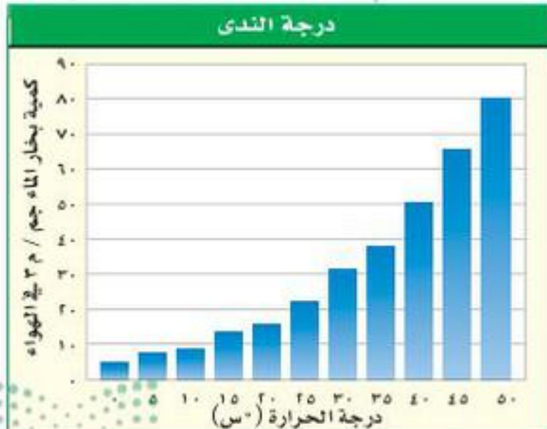
الشكل ٧ يوضح الشكل تأثير درجة الحرارة في كمية بخار الماء التي يستطيع الهواء حملها. حدد مقدار بخار الماء الذي يستطيع الهواء حمله، إذا كانت درجة حرارته ٣٠°س، و ١٠°س، على التوالي.
