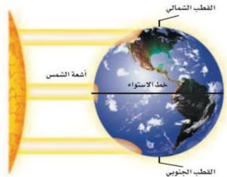
الشكل ١٠ تكون زاوية سقوط أشعة الشمس كبيرة عند خط الاستواء، وصغيرة عند القطبين.
